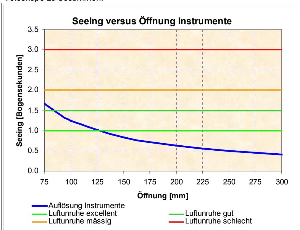
Abb. 8: Bestimmen der notwendigen minimale Öffnung des Teleskops in Abhängigkeit vom Seeing.
