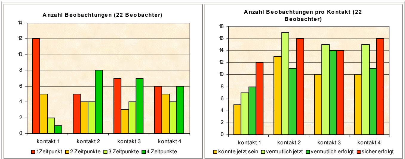
Abb. 4: Anzahl Beobachtungen
