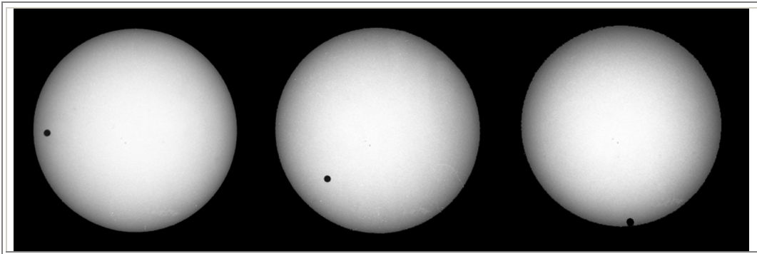
Abb. 2: Der Venustransit vom 8. Juni 2004
